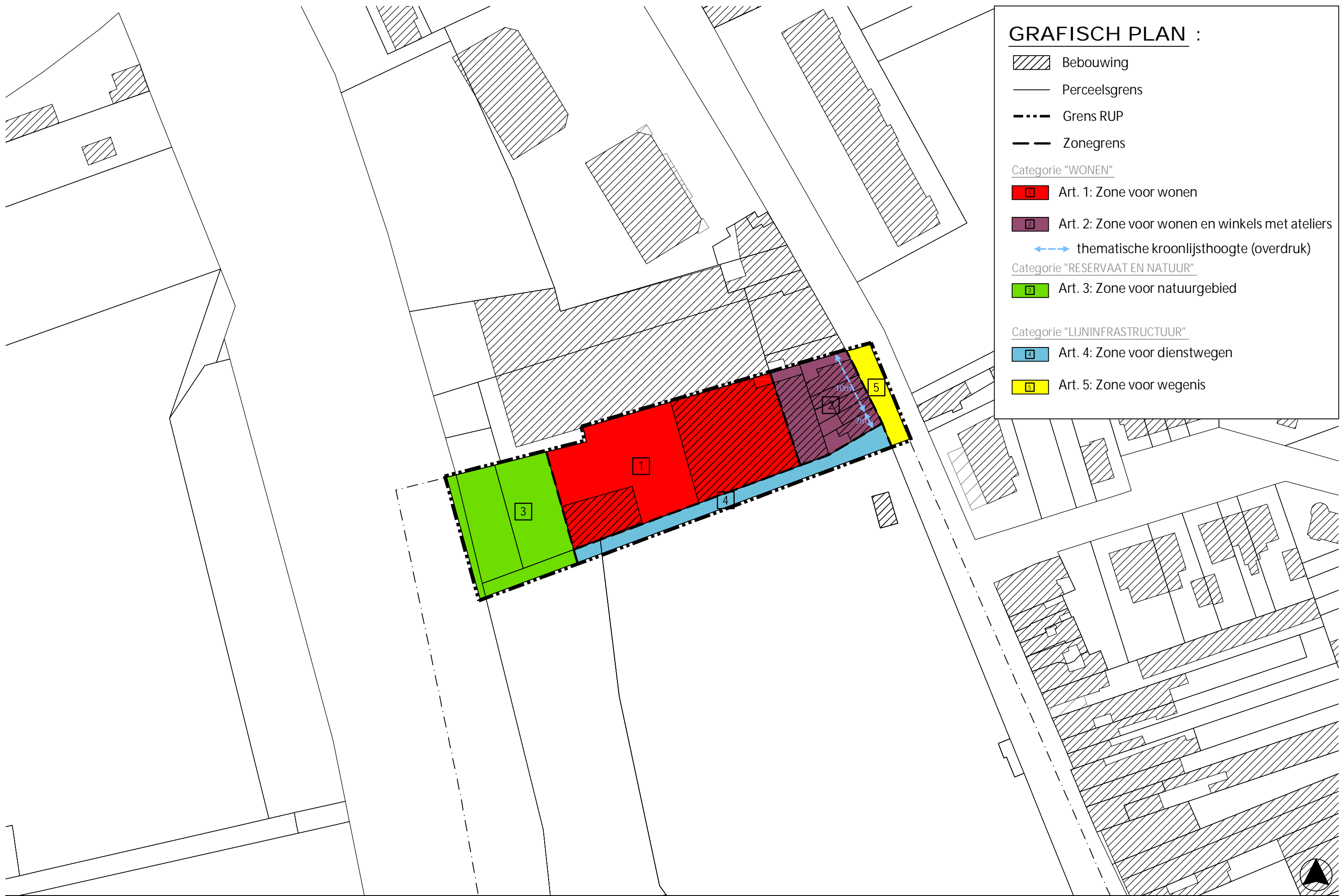
GRAFISCH PLAN (1/1.000)
